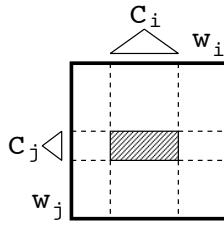
図 2: w_i, w_j ともに抽象化した場合
