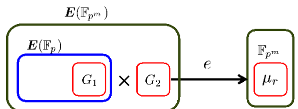
【図3 楕円曲線を用いた新暗号系の基本写像】
