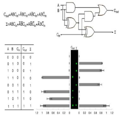
図1 独自に開発した光で駆動するDNA論理回路を用いた自律的なDNA計算
