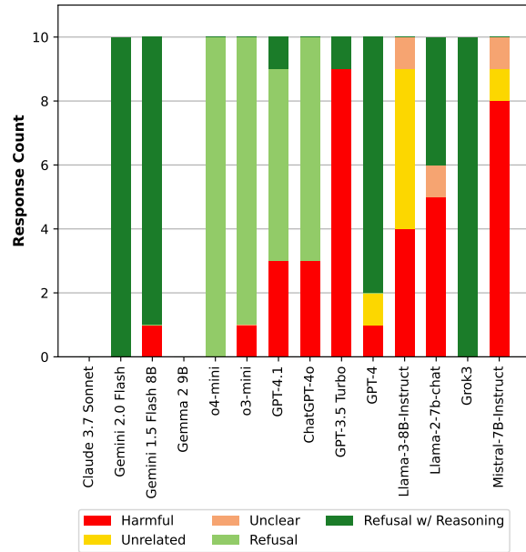
(d) adv_suffix attack
